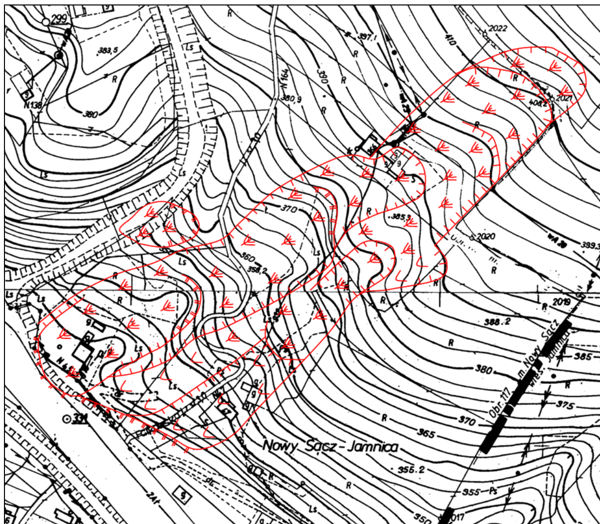
Szkic osuwiska na mapie zasadniczej w skali 1 : 2000
