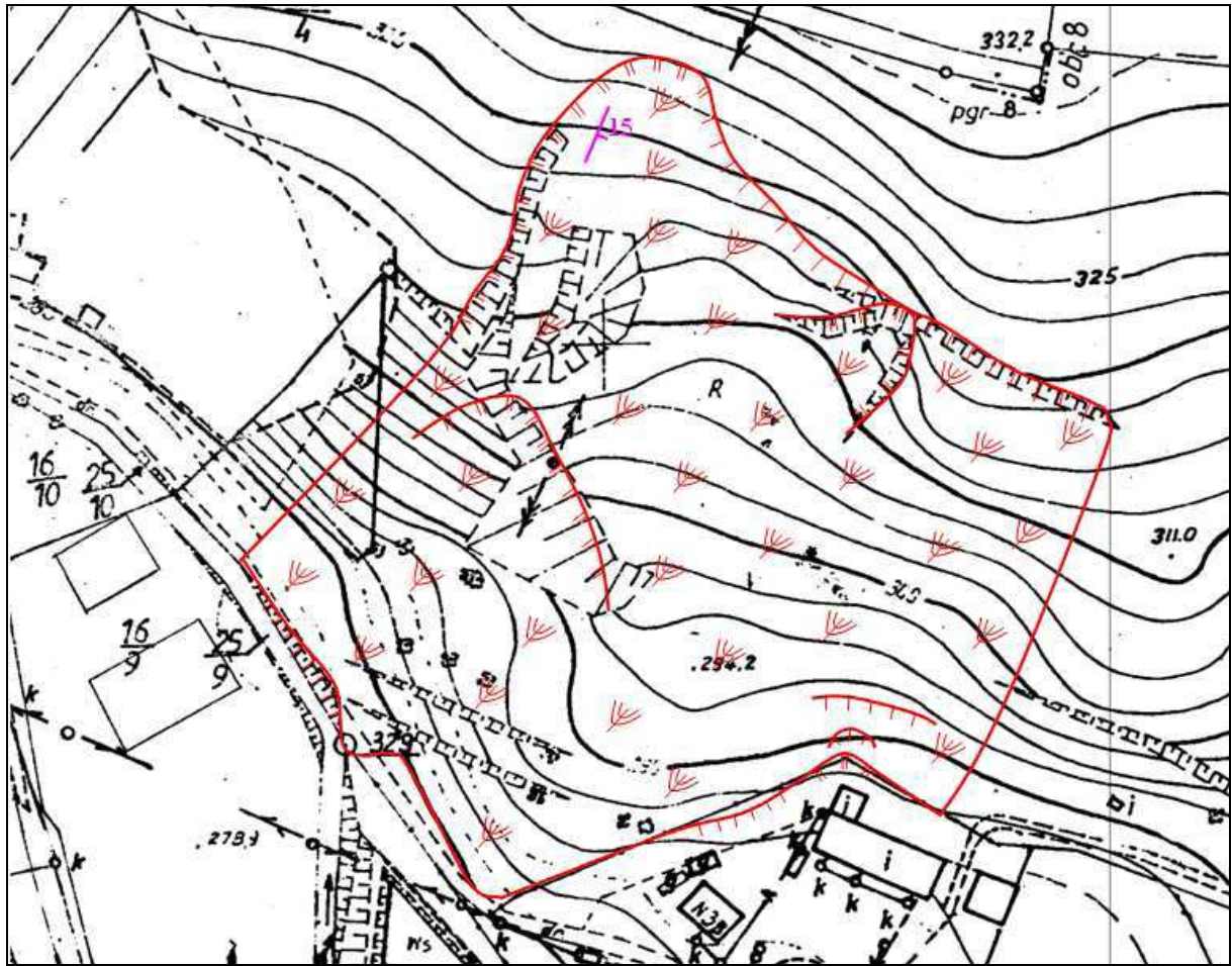
Szkic osuwiska na mapie zasadniczej w skali 1 : 2000
