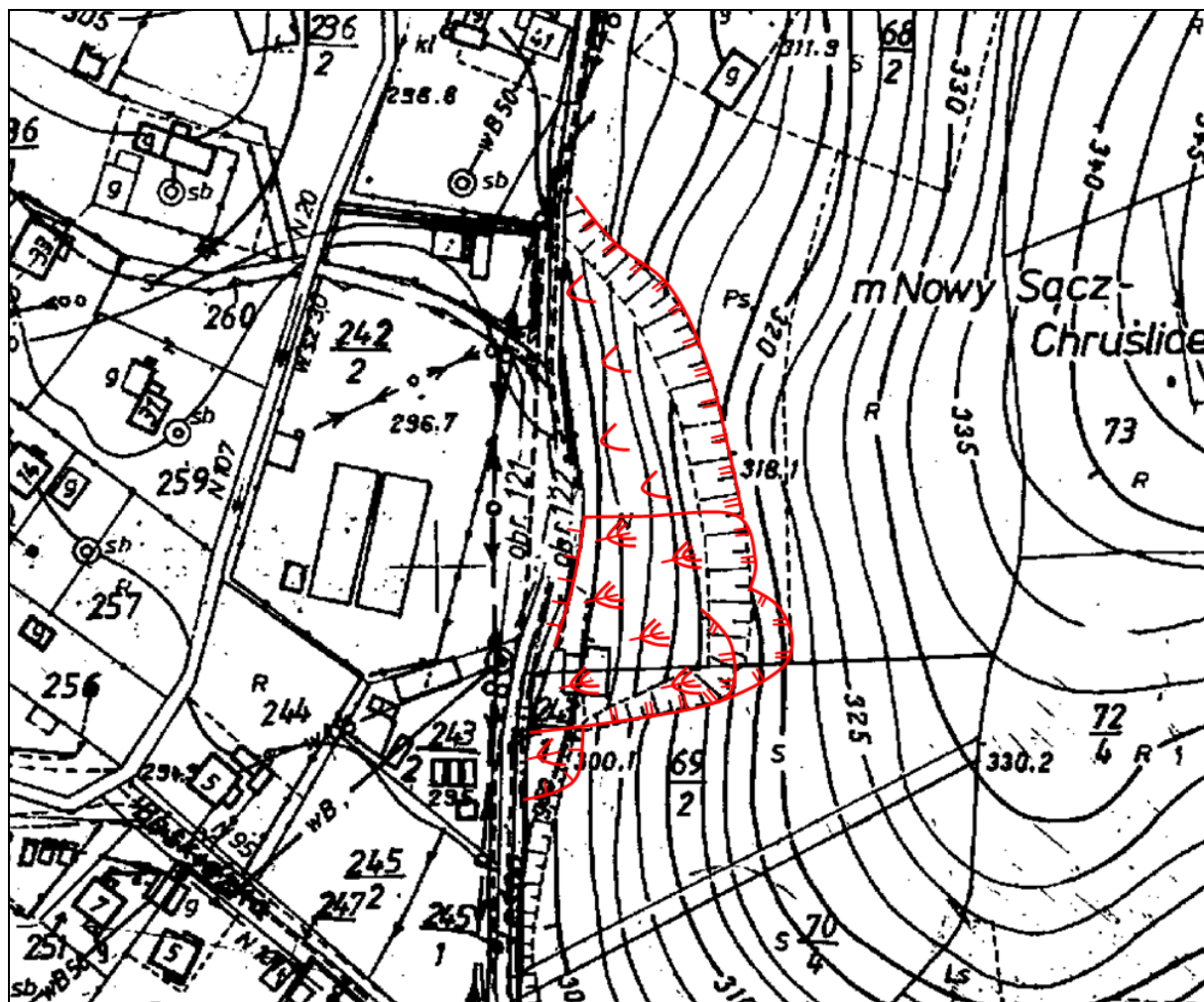
Szkic osuwiska na mapie zasadniczej w skali 1 : 2000
