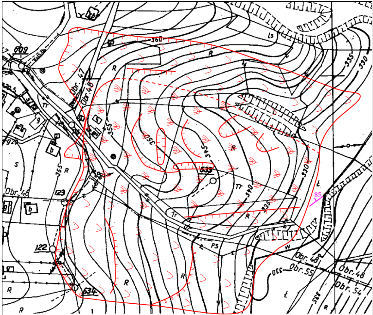
Szkic osuwiska na mapie zasadniczej w skali 1 : 2000
